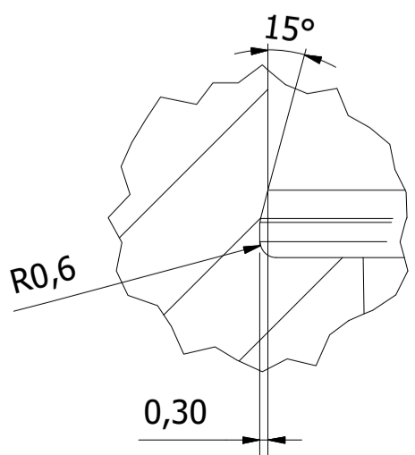
DETTAGLIO SCARICO CUSCINETTO
